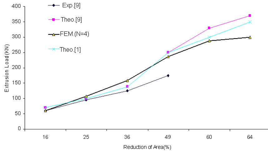
شکل ۱: تاثير درصد کاهش سطح مقطع بر بار اكستروژن برای بيلت مربعی، سنجه دایروی و m=0.1 .
