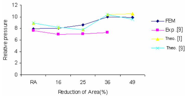
شکل ۲: تاثير درصد کاهش سطح مقطع بر فشار نسبی برای بيلت مربعی، سنجه دایروی و m=0.1 .
